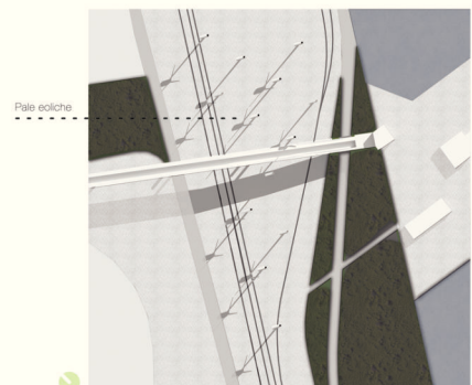
Planivolumetrico Sezione D - D' Scala 1:2000
