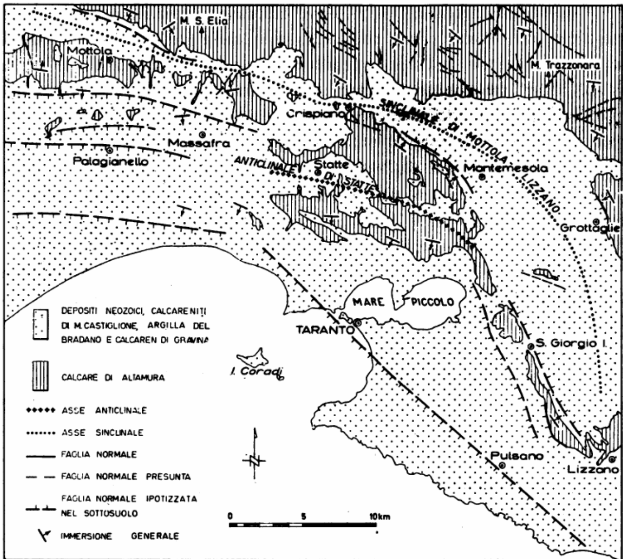
Fig. 16.2 – Schema tettonico dell'area di Taranto.
